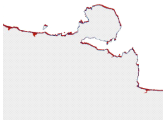
Χάρτης απεικόνισης των παράκτιων περιοχών που θα ατακλυστούν (κόκκινο χρώμα) από ενδεχόμενη άνοδο της θάλασσας στάθμης κατά 2 μέτρα, μέχρι το 2100.
